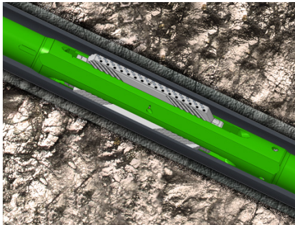
Дизайн секционного фрезера системы ProMILL Duo позволяет проходить через обсадную колонну меньшего диаметра с последующим фрезерованием как внутренней, так и внешней колонны.
