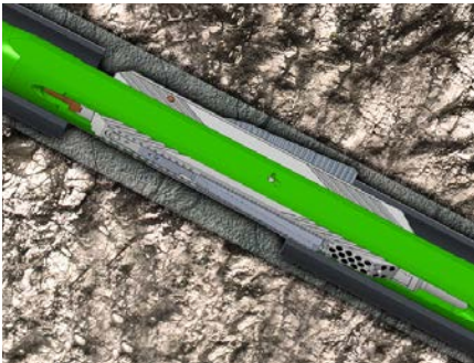
Система состоит из секционного фрезера с выдвижными лопастями расширенного диапазона и гидравлического стабилизатора, для обеспечения эффективного фрезерования при ликвидации скважин в интервалах с двойной обсадной колонной.
