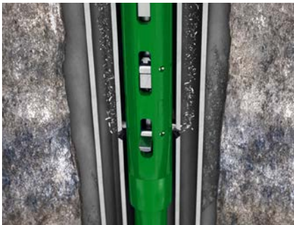
Многоцикличный труборез позволяет производить многочисленные прорезания колонны за один спуск, сокращая при этом операционное время и уменьшая риски инцидентов, связанных с дополнительной работой на столе ротора буровой бригады.
