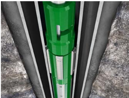
Когда труболовка системы ProCISE в положении захвата с колонной, производится тест натяжением вверх. При успешном тесте, когда сцепление подтверждено, производится прорезание обсадной колонны в натяжке (для ускорения процесса).
